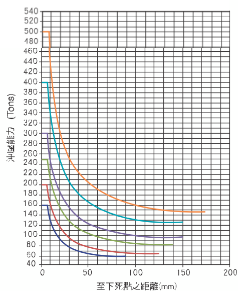
行程-能力曲線圖(S)
