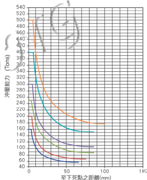
行程-能力曲線圖(H)
