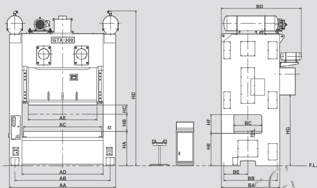
外觀尺寸 (A型)
