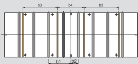
Fig. 4 圖形四(含舉模器用"U"型溝)
